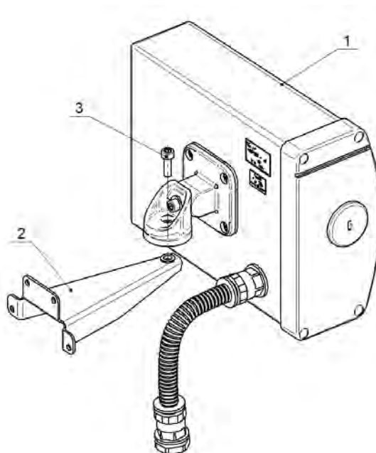
Рисунок 2.8 – Установка блока ПРД (блока ПРМ) на кронштейне 120М
